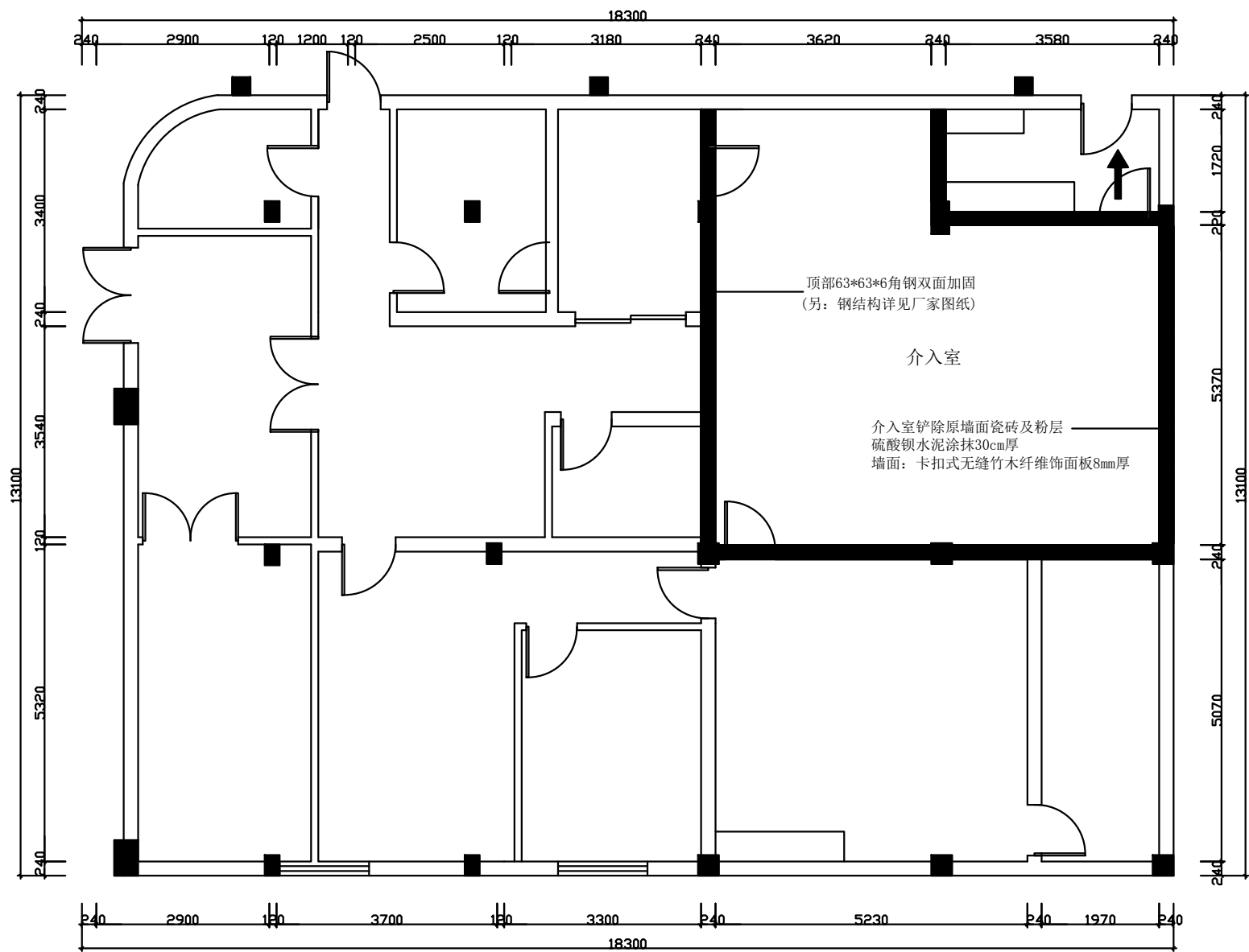
襄阳市第一医院墙面处理图
