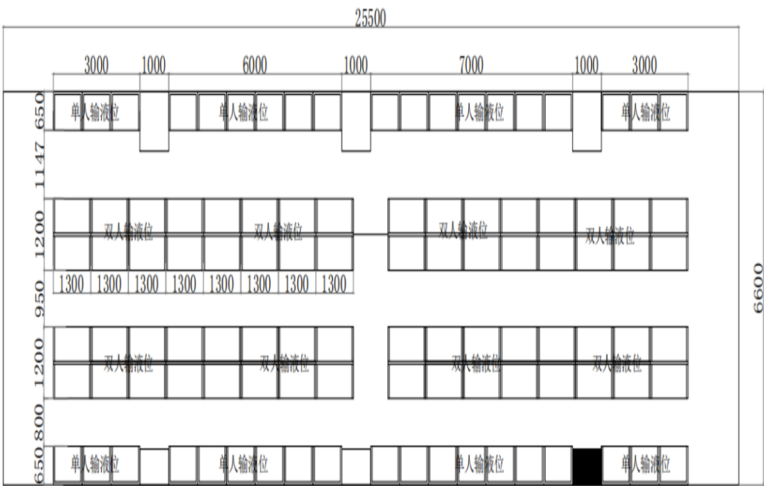
儿童输液室平面布置图
