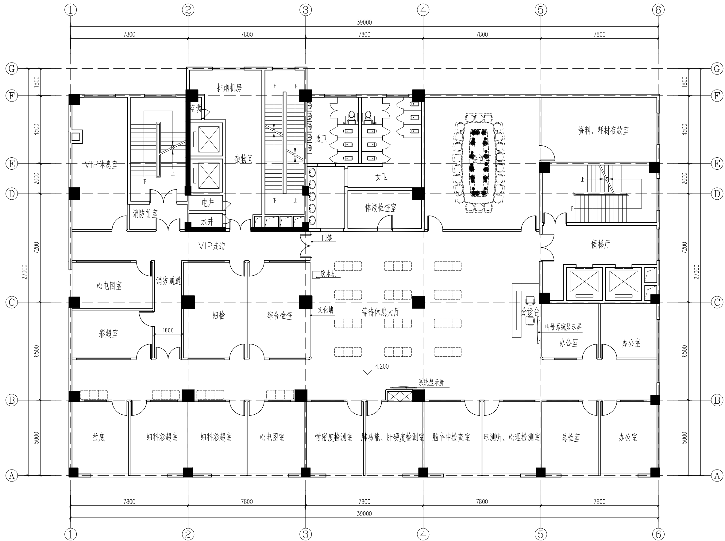
改造后二层平面图 1:100 本层建筑面积 1010.08m 2
